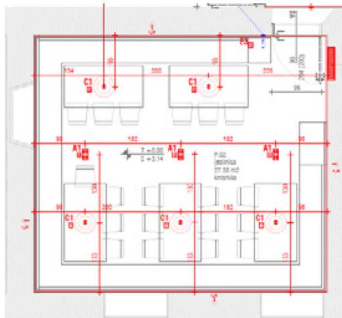
Načrt druge jedilnice
