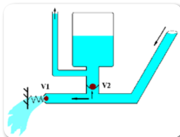
Shema delovanja hidravličnega ovna
